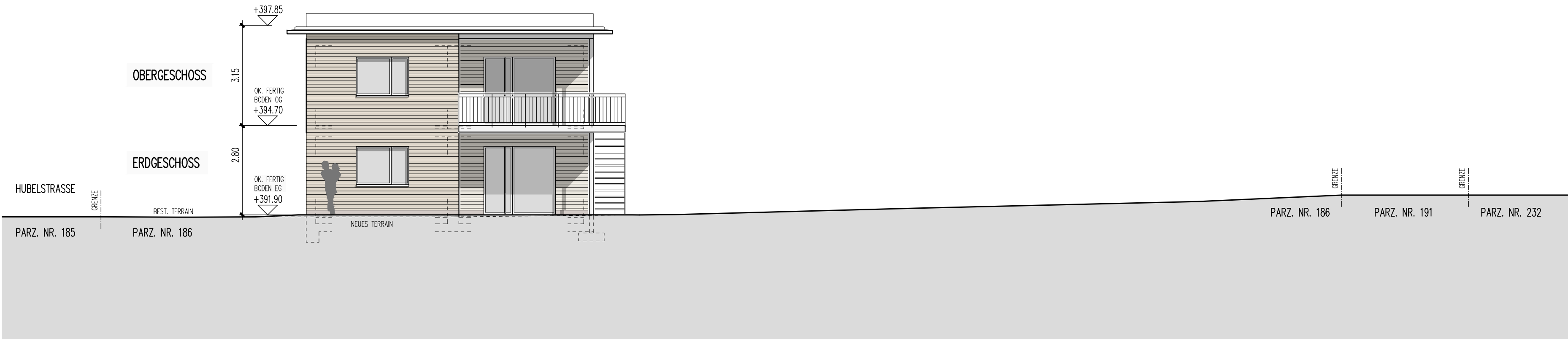
SÜDWEST – FASSADE
