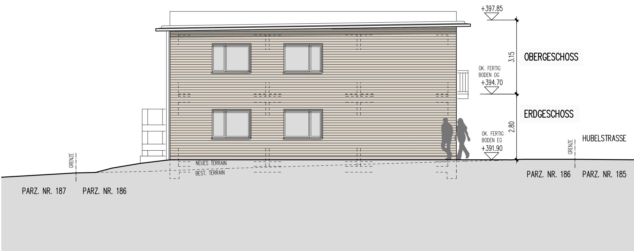
NORDWEST – FASSADE
