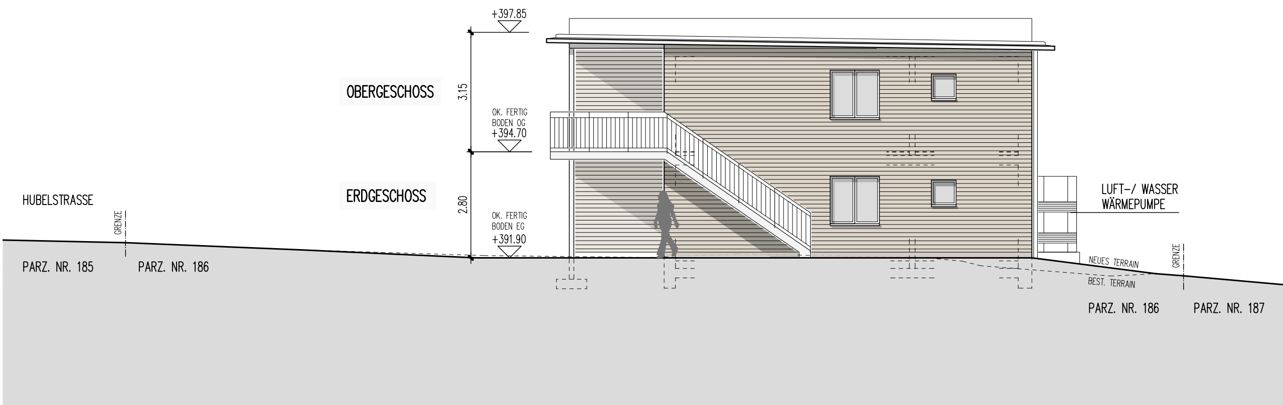
SÜDOST – FASSADE
